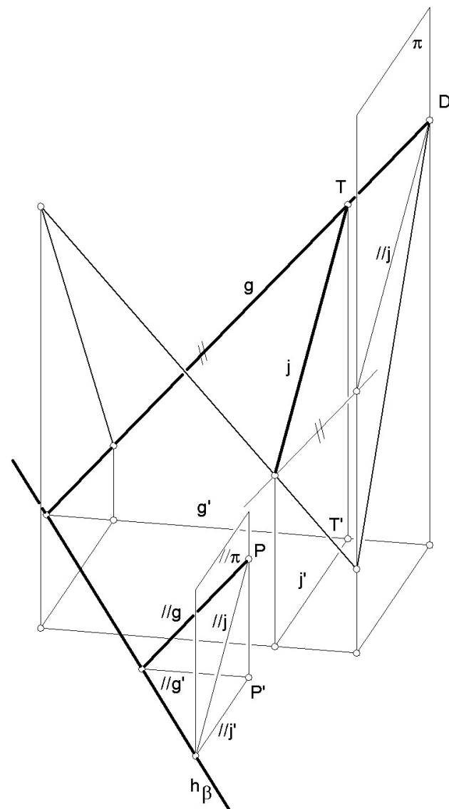
PLANO TANGENTE CONDUZIDO POR UM PONTO EXTERIOR
