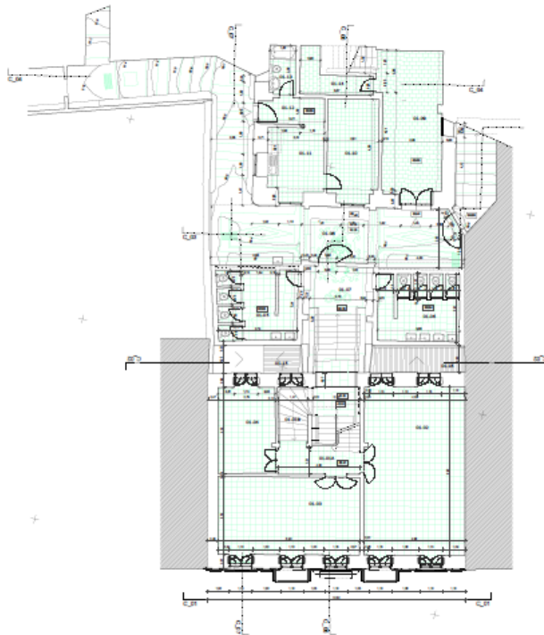
Planta 1
