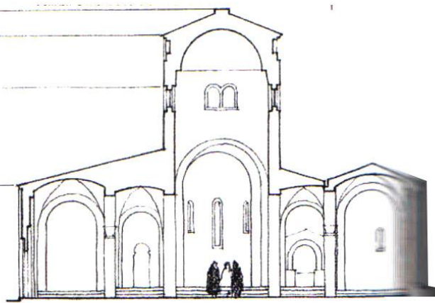
Corte transversal
