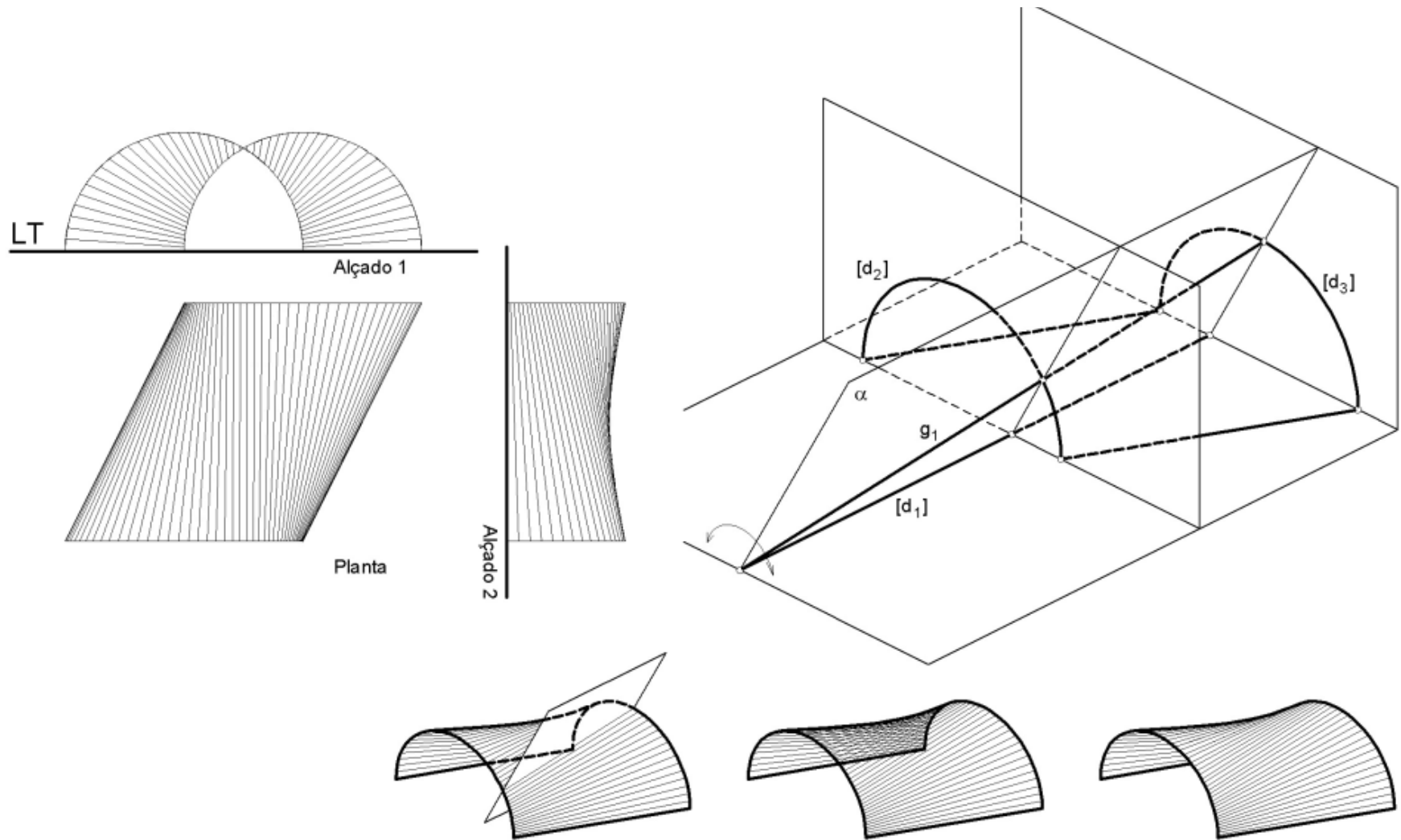
SUPERFÍCIE DE ARCO ENVIESADO - "CORNO DE VACA"
