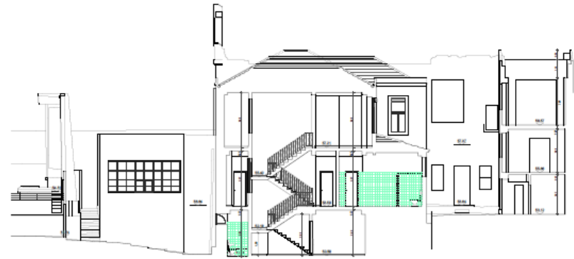
Corte 04
