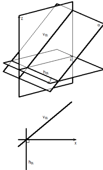
PLANO DE TOPO
