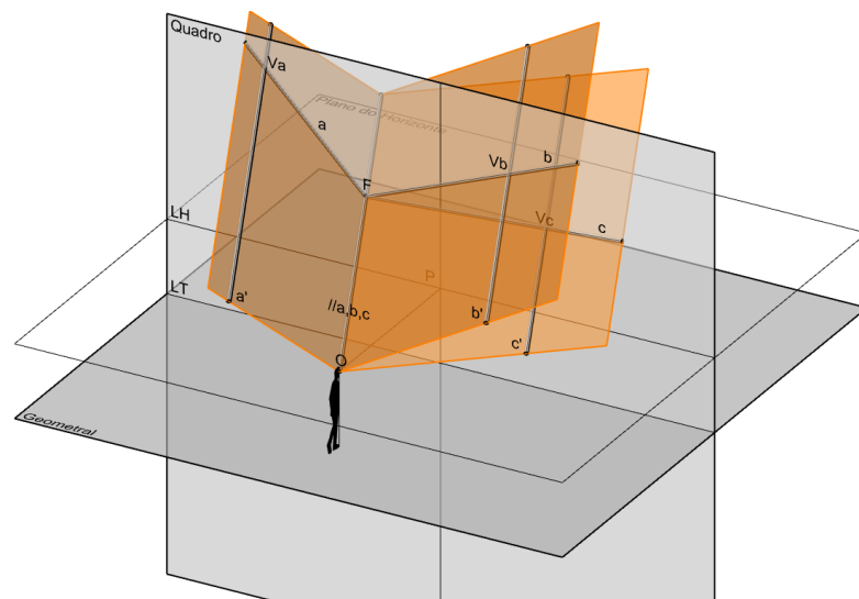
Rectas oblíquas (Pontos de fuga exteriores à vertical passante por P e à LH)
