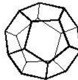
Dodecaedro
