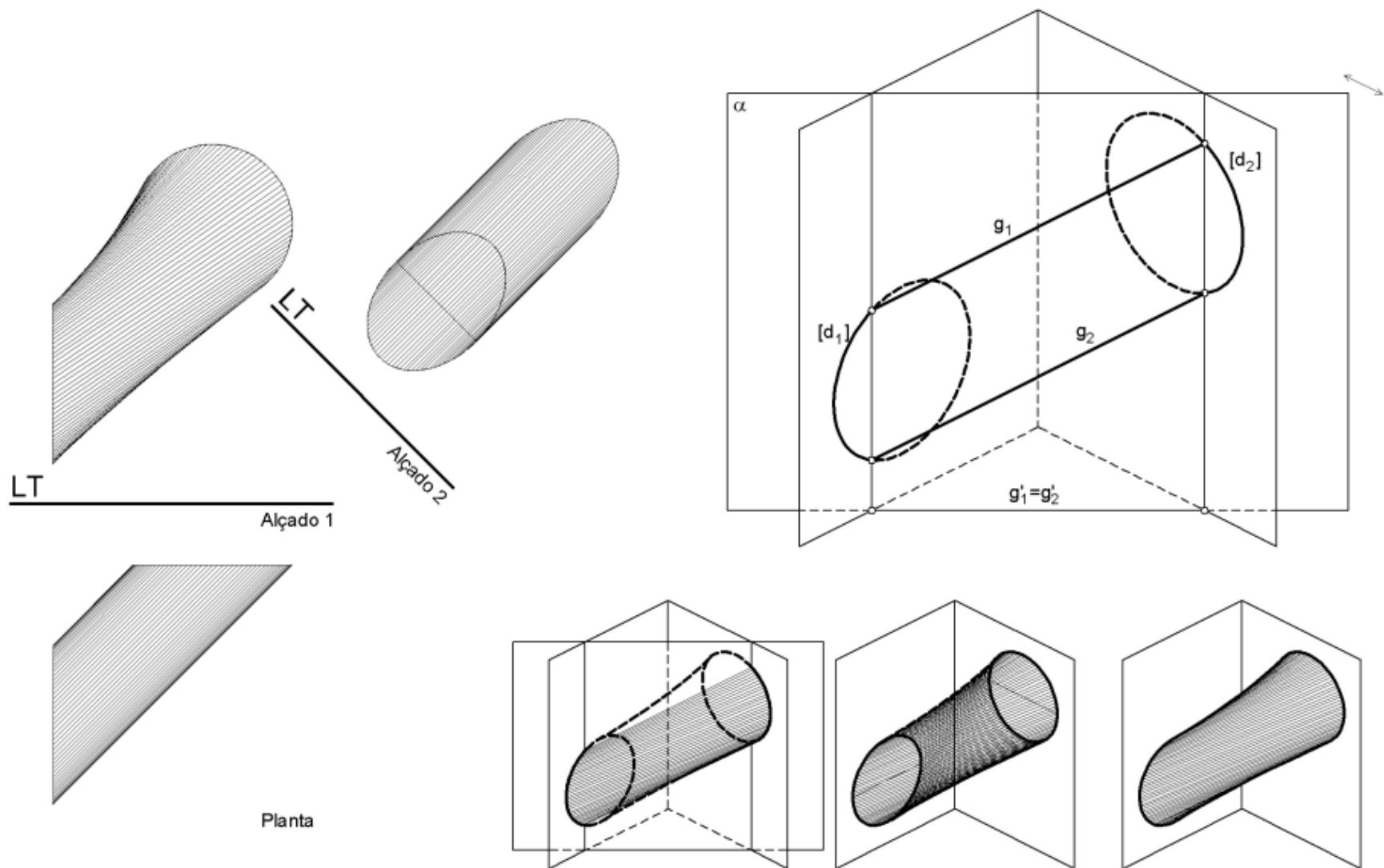
SUPERFÍCIE DE CILINDRÓIDE DE DIRECTRIZES CIRCUNFERENCIAIS
