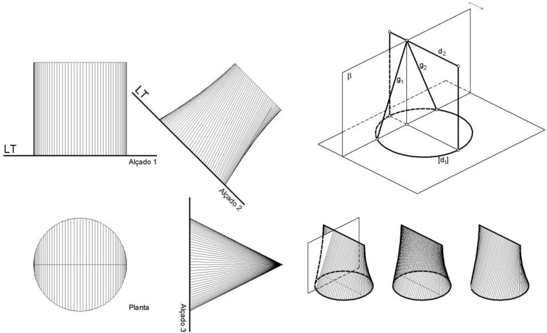
SUPERFÍCIE DE CONÓIDE RECTO DE DIRECTRIZ CIRCUNFERENCIAL
