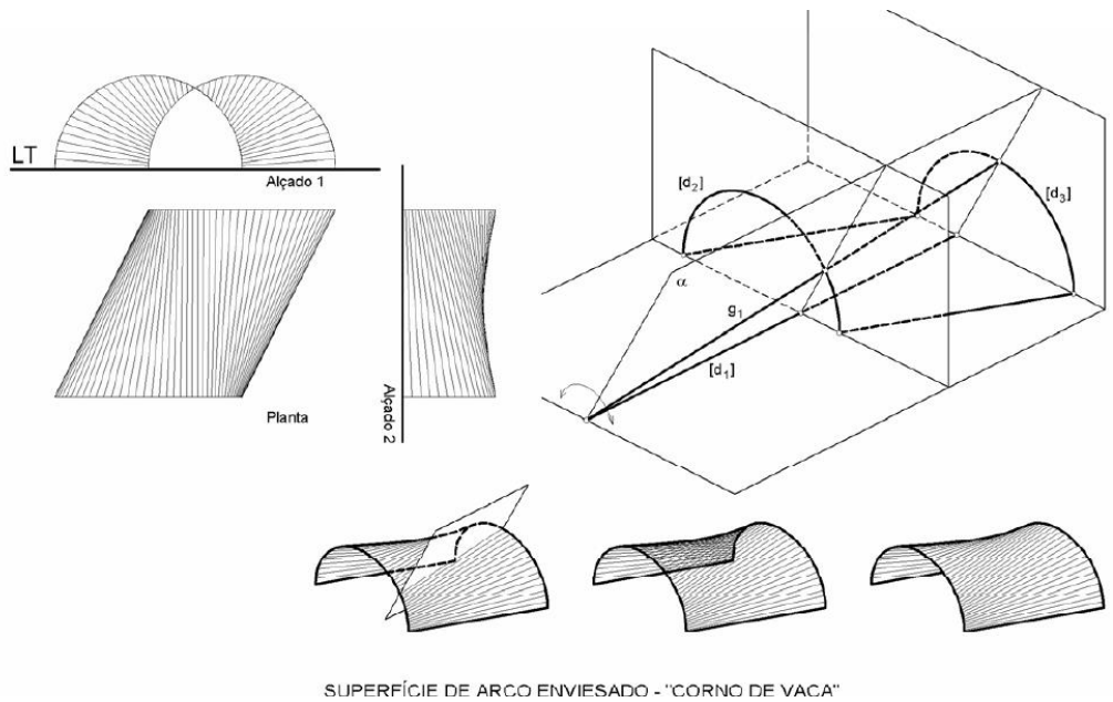
SUPERFÍCIE DE ARCO ENVIÉSADO - "CORNO DE VACA"
