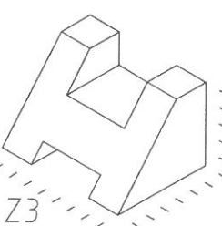
Figura 4.64 - Exercícios de projeção de peças (continuação).
