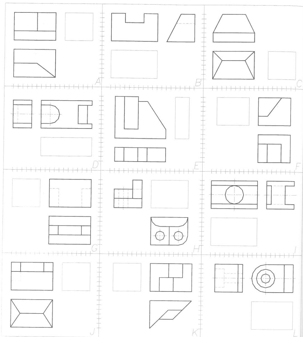
Figura 4.65 - Exercícios para completar a terceira projecção (continua).
