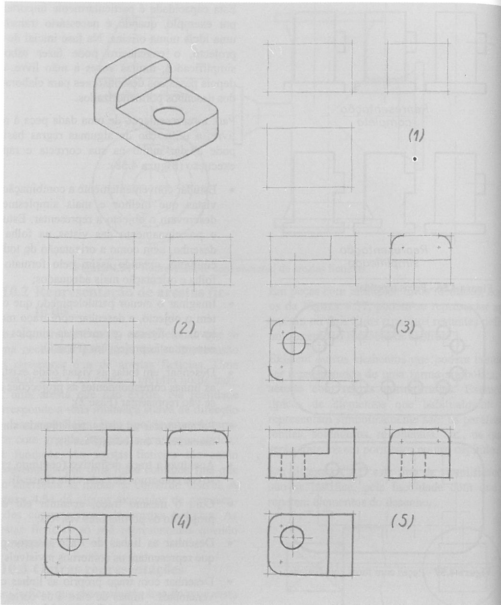
Figura 4.58 - Fases de construção de um desenho à mão livre.
