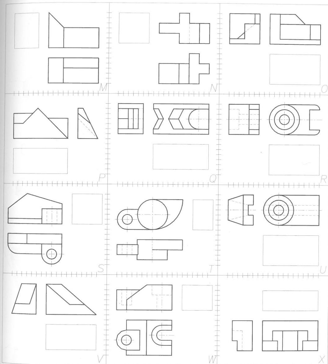
Figura 4.65 - Exercícios para completar a terceira projecção (continuação).
