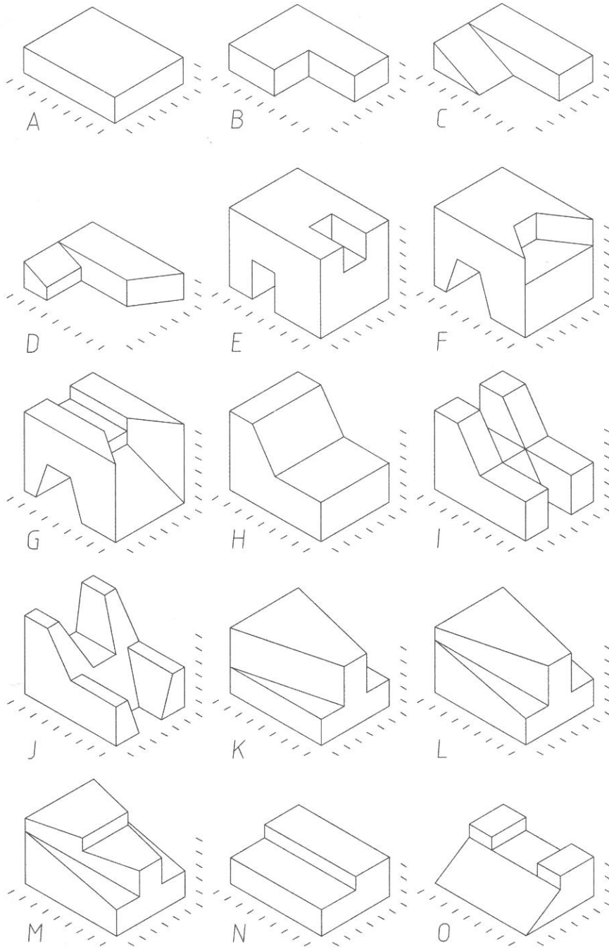
Figura 4.64 - Exercícios de projecção de peças (continua).
