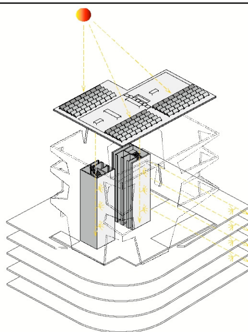
PAINÉIS FOTOVOLTAICOS energia solar para iluminação das colunas de escadas e dos pisos de estacionamento
