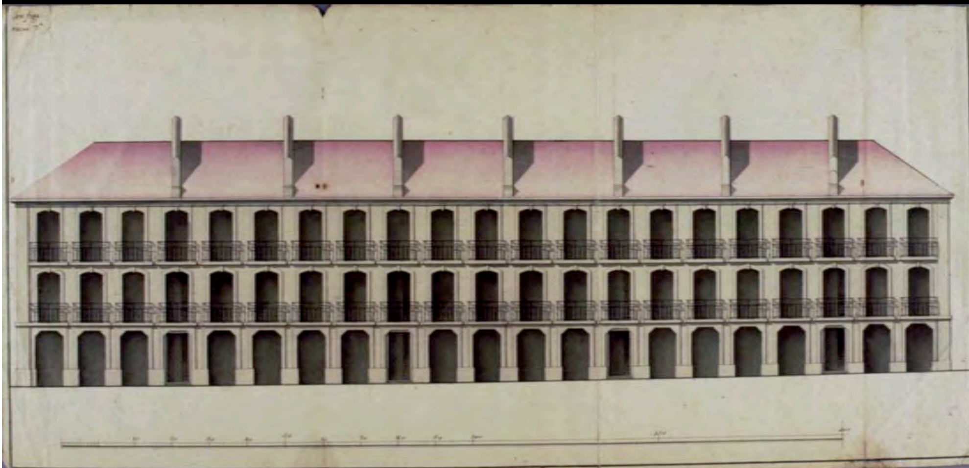
Desenho para fachada tipo anexo à Dissertação de Manuel da Maia, Eugénio dos Santos, 1756 — MC(L)
