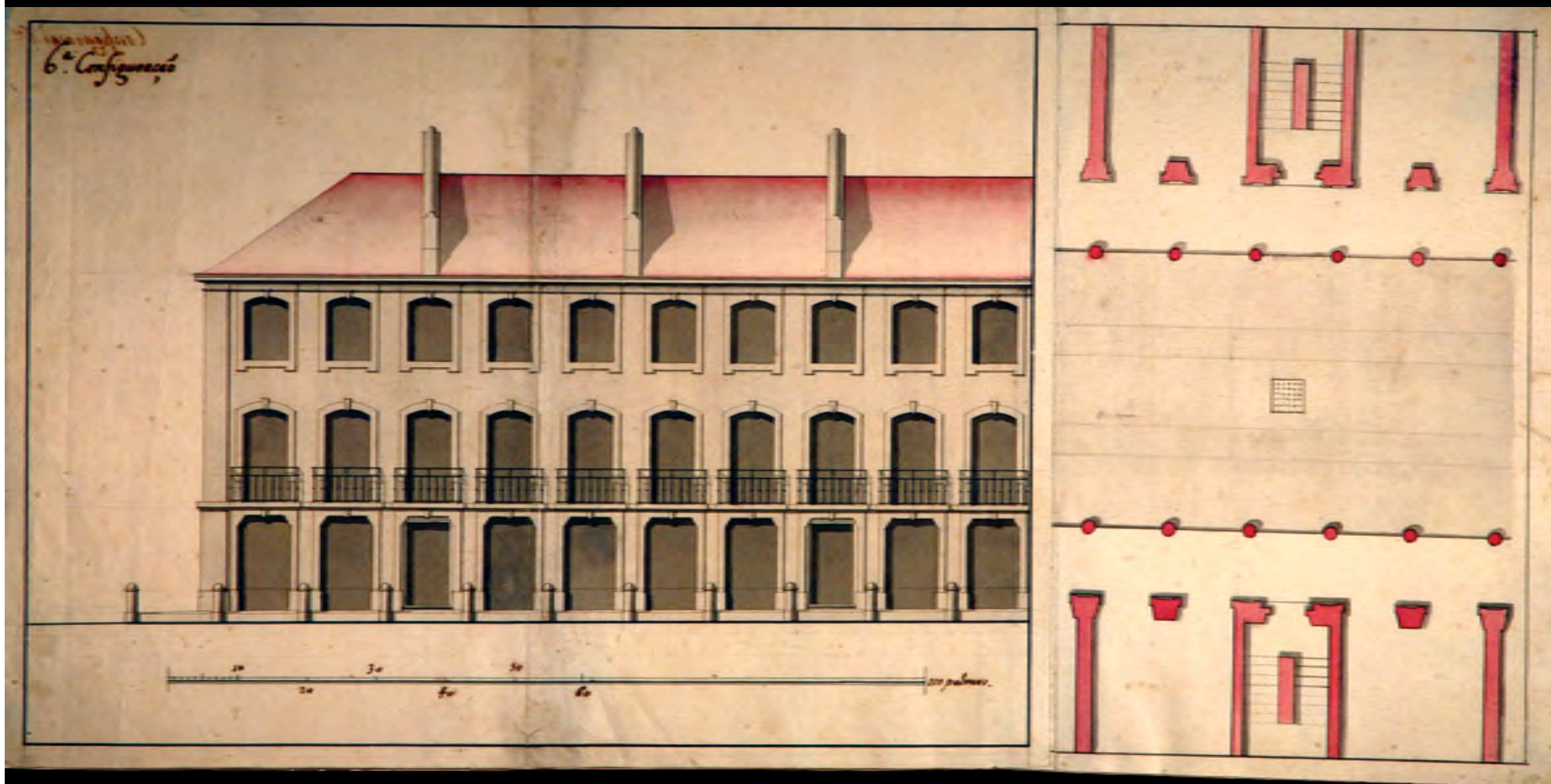
Desenhos para fachada tipo anexos à Dissertação de Manuel da Maia, Eugénio dos Santos, 1756 — MC(L)
