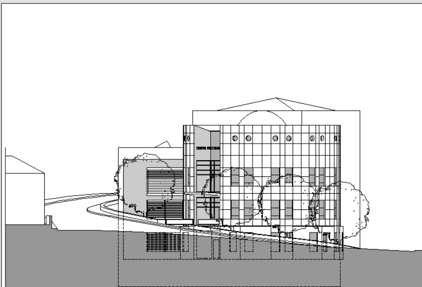
Alçado Norte escala 1:300
