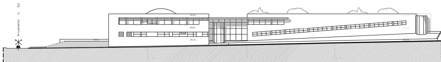
ALÇADO NASCENTE
