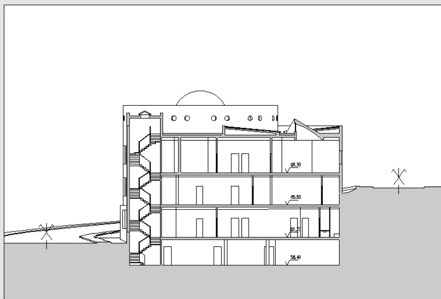
Corte BB' escala 1:300
