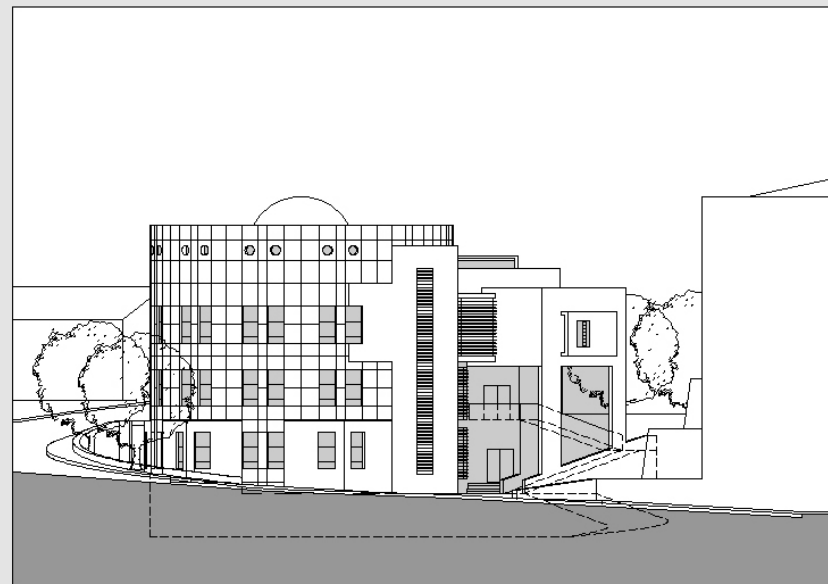
Planta Poente escala 1:300
