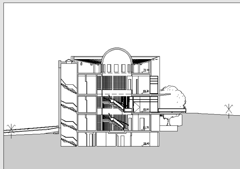
Corte AA' escala 1:300
