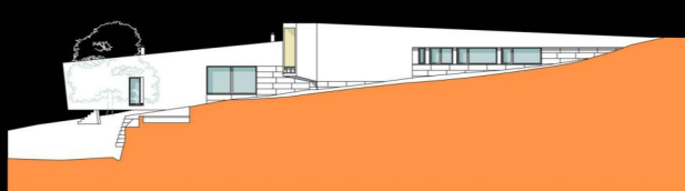
ALÇADO NORDESTE
