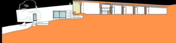
CORTE LONGITUDINAL
