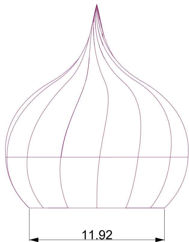
Alçado frontal 1/20
