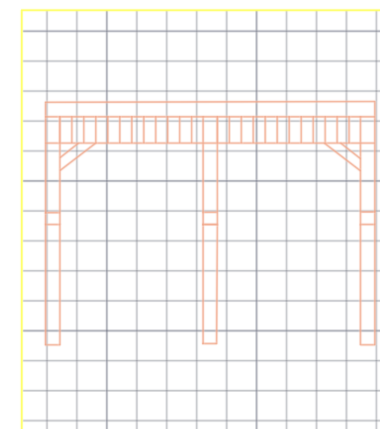
ALCADO 3 1/50
