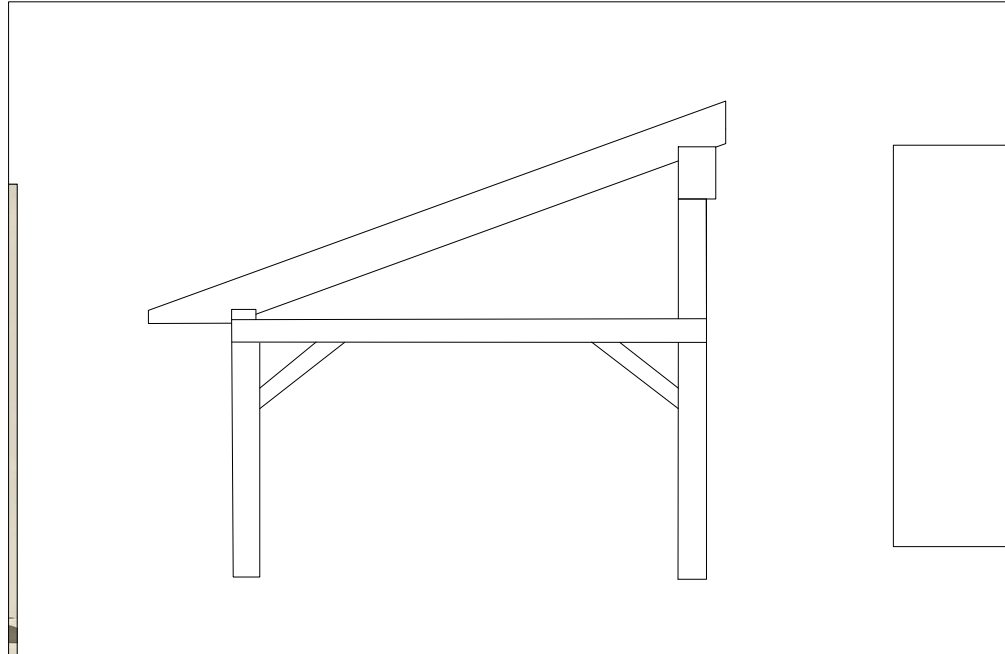
Alçado lateral
