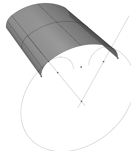
ABÓBADA ABATIDA CONSTRUÍDA NO GRASSHOPPER
