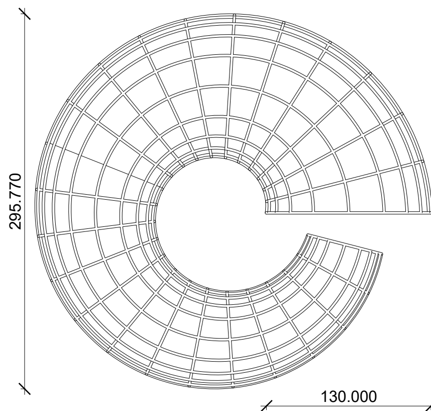
VISTA DE TOPO
