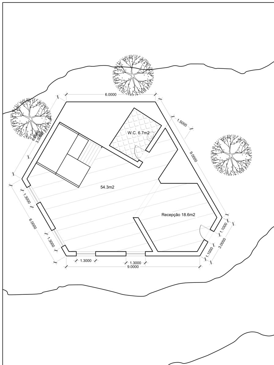
planta 1/100
