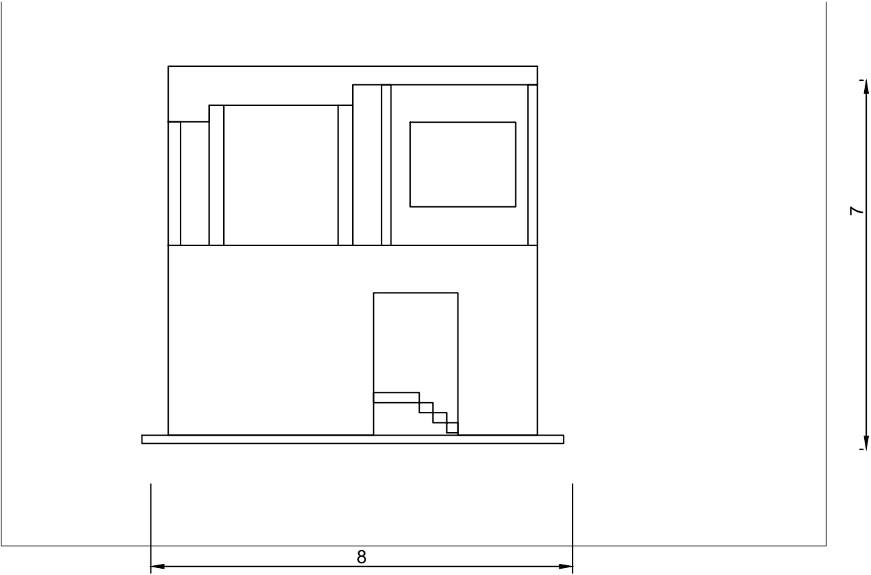
Alçado frontal 1:100
