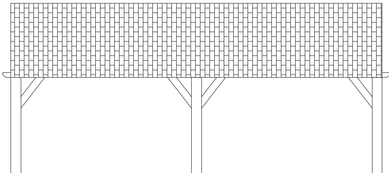
Alçado lateral 1:50
