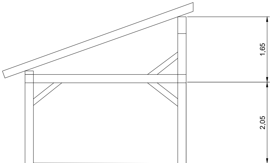
Alçado lateral 1:50
