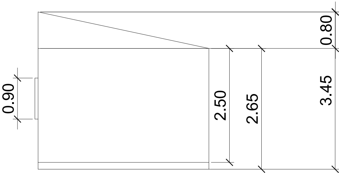
Alçado Oeste
