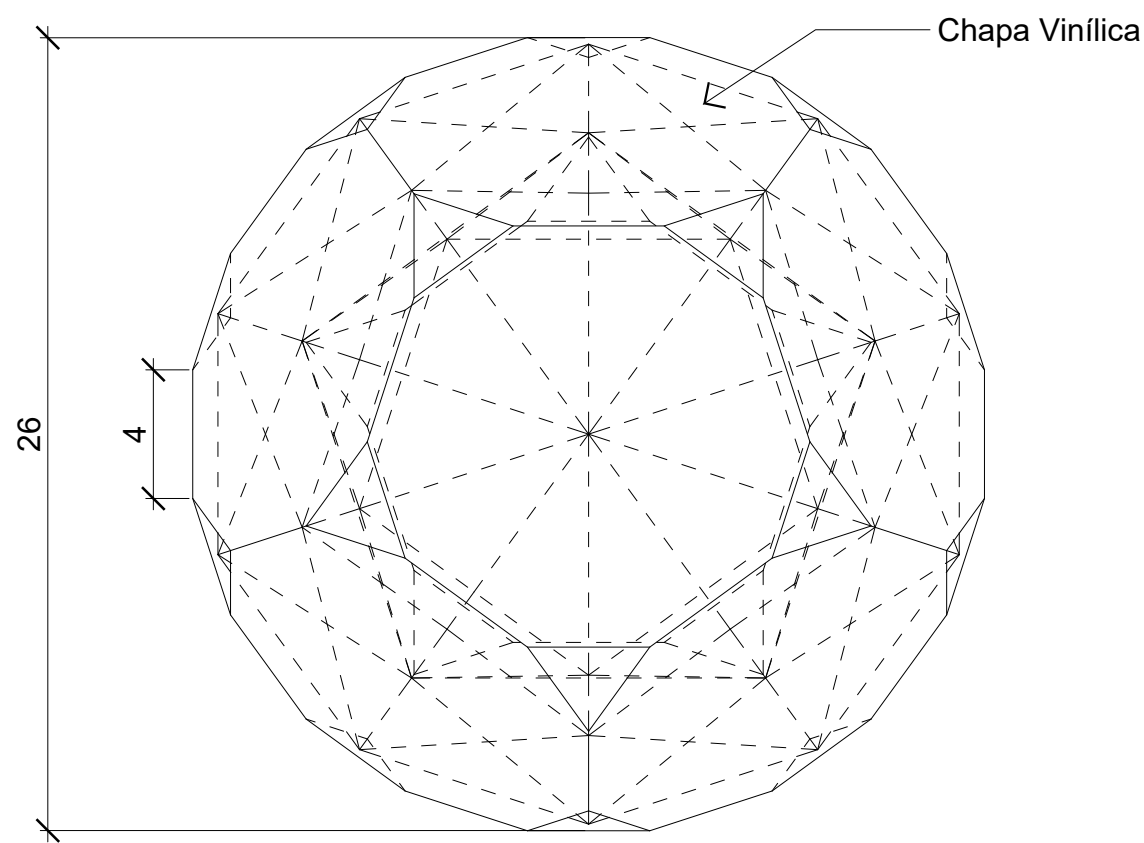
Planta 1:4
