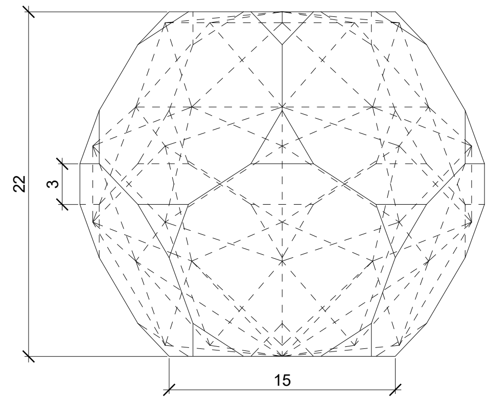
Alçado Frontal 1:4
