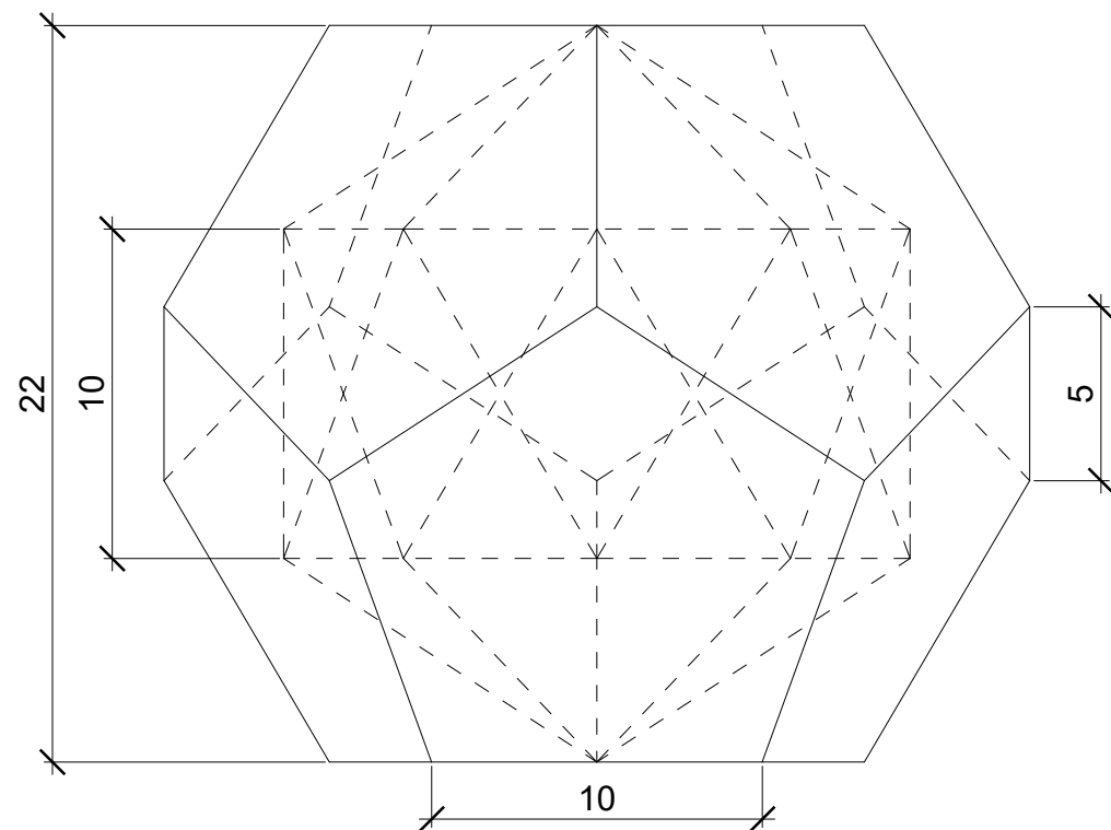
Alçado Frontal 1:4
