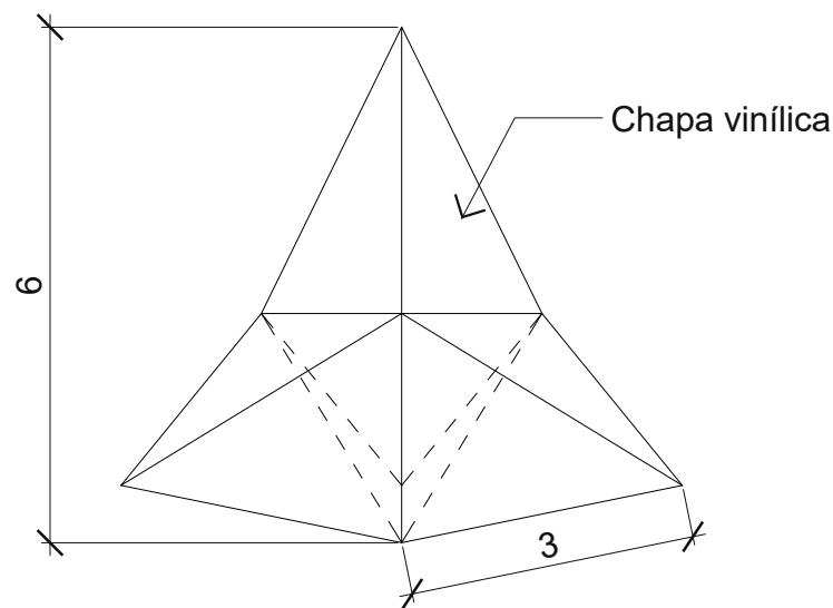
Alçado Frontal 1:1
