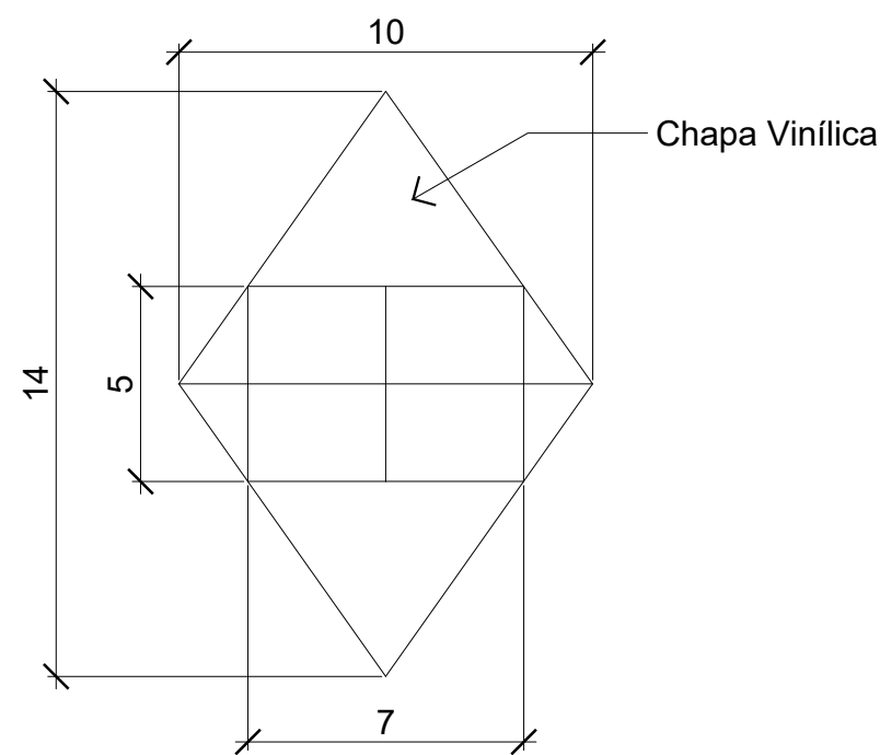
Alçado Frontal 1:2
