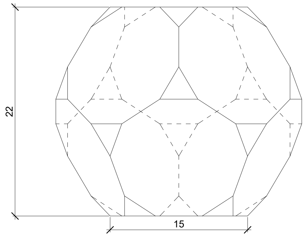
Alçado Frontal 1:4
