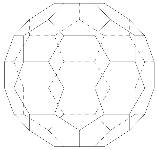
Alçado Frontal
