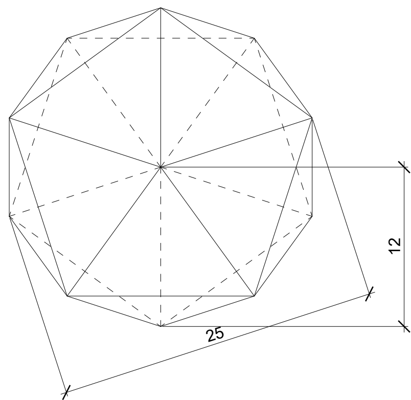
Planta 1/4
