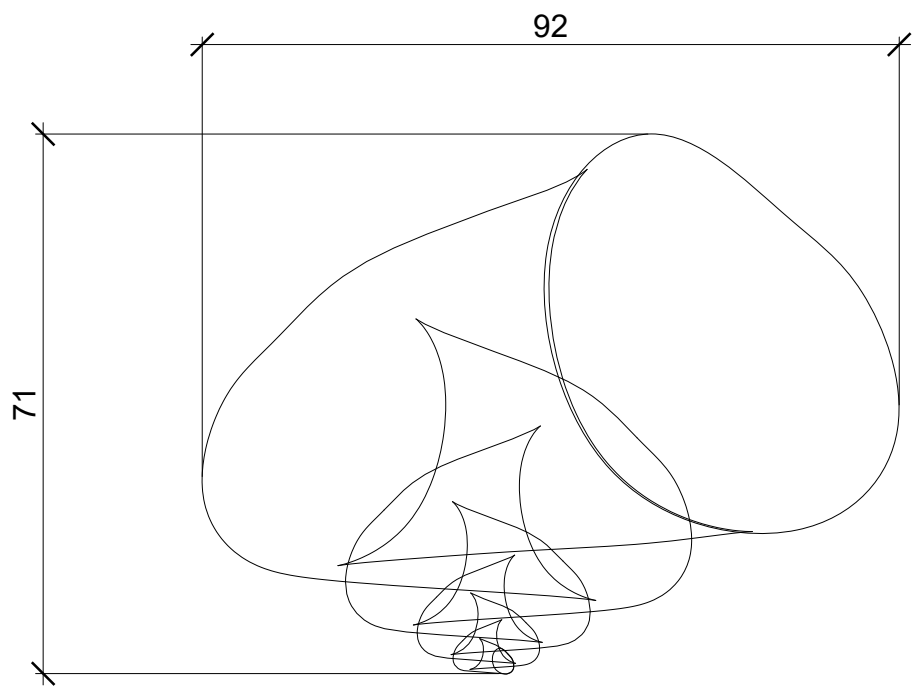
Alçado Frontal 1:1
