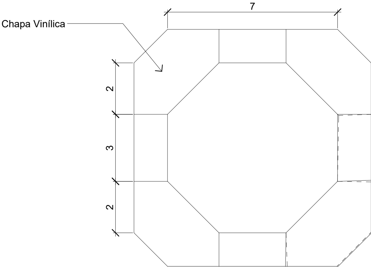
Planta 1:1
