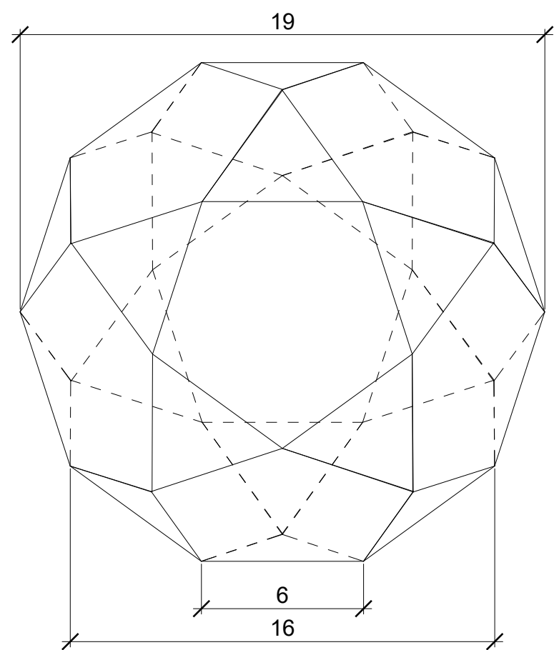
Planta 1:5
