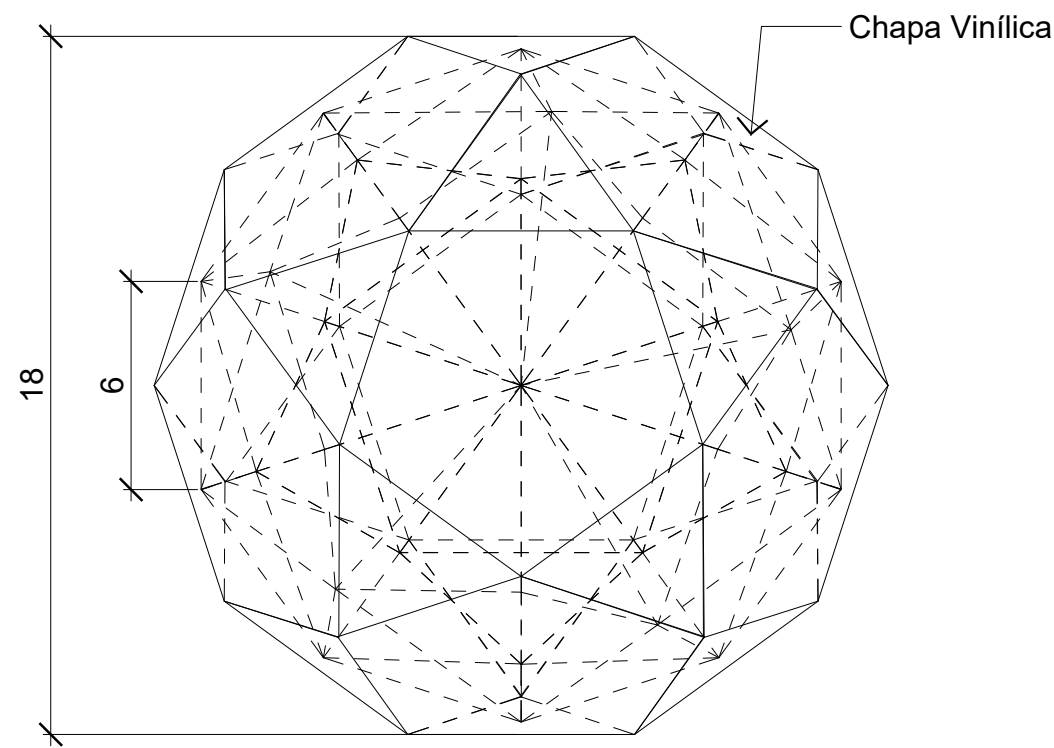
Planta 1:5
