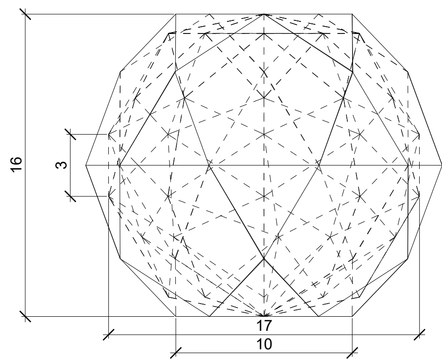
Alçado Frontal 1:5
