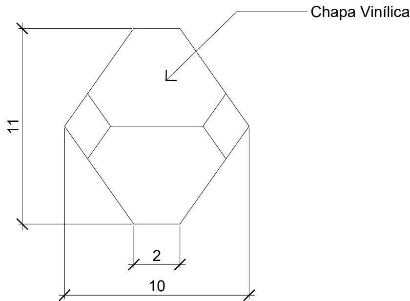
Alçado Frontal 1:2
