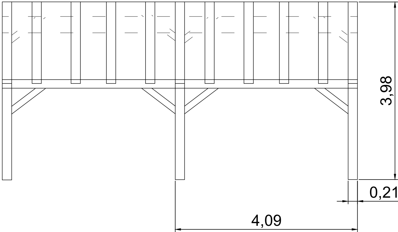
Alçado Frontal 1/50
