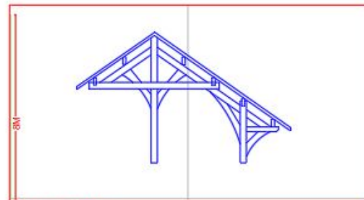
ALÇADO LATERAL 1/50
