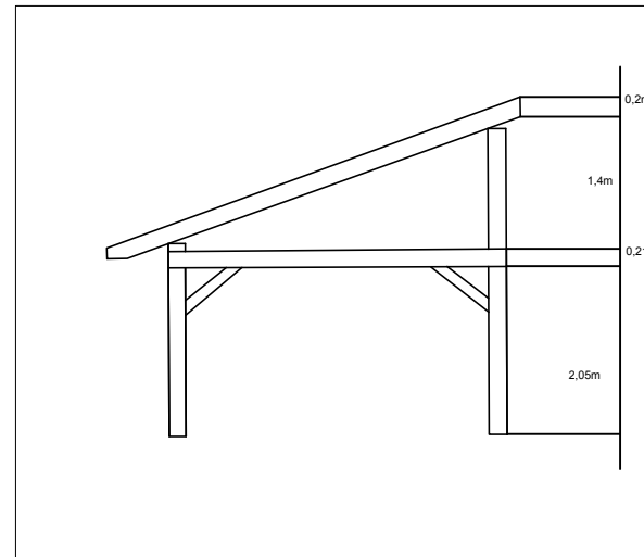
alçado 1:100
