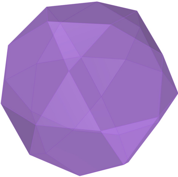
Icosidodecaedro
