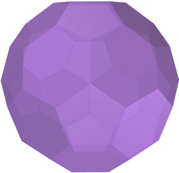
Icosaedro Truncado
