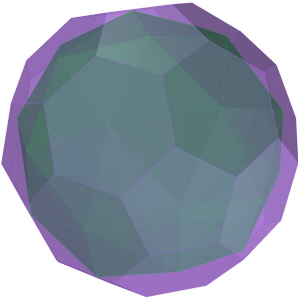
Icosaedro Truncado e Dual
