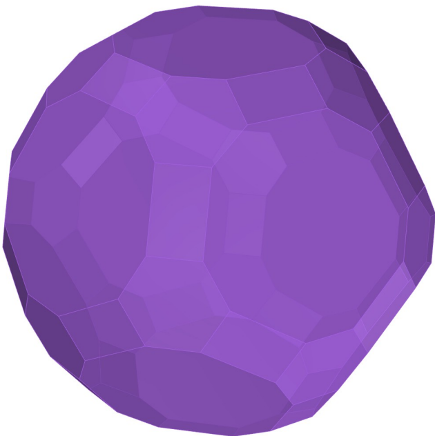
Icosidodecaedro Truncado
