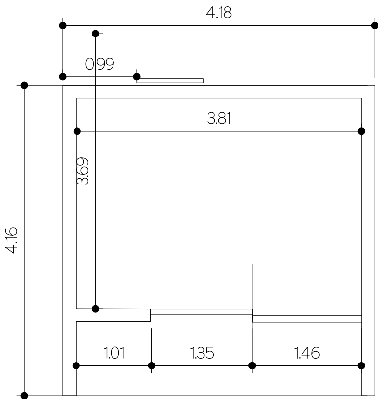
Planta
