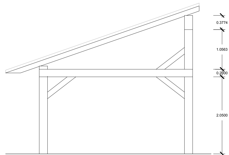
ALÇADO ESC. 1/50
