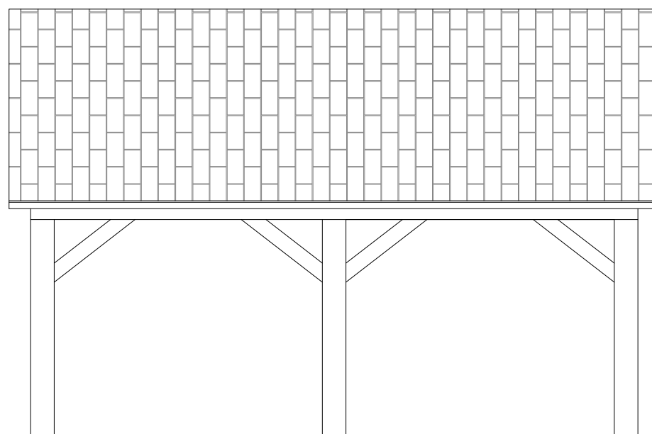
ALÇADO ESC. 1/50
