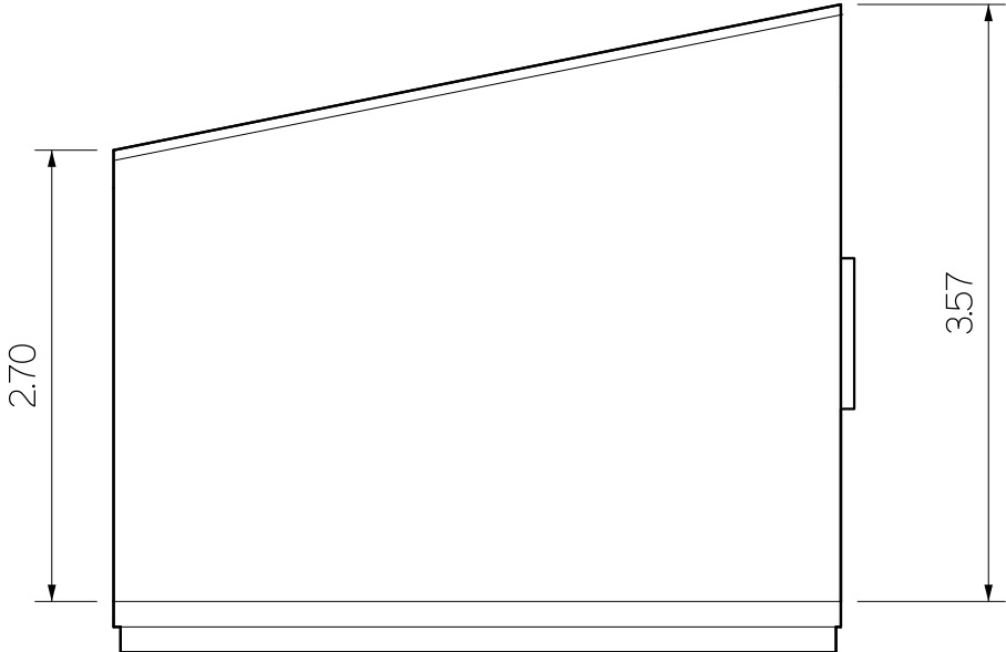
Alçado Este
