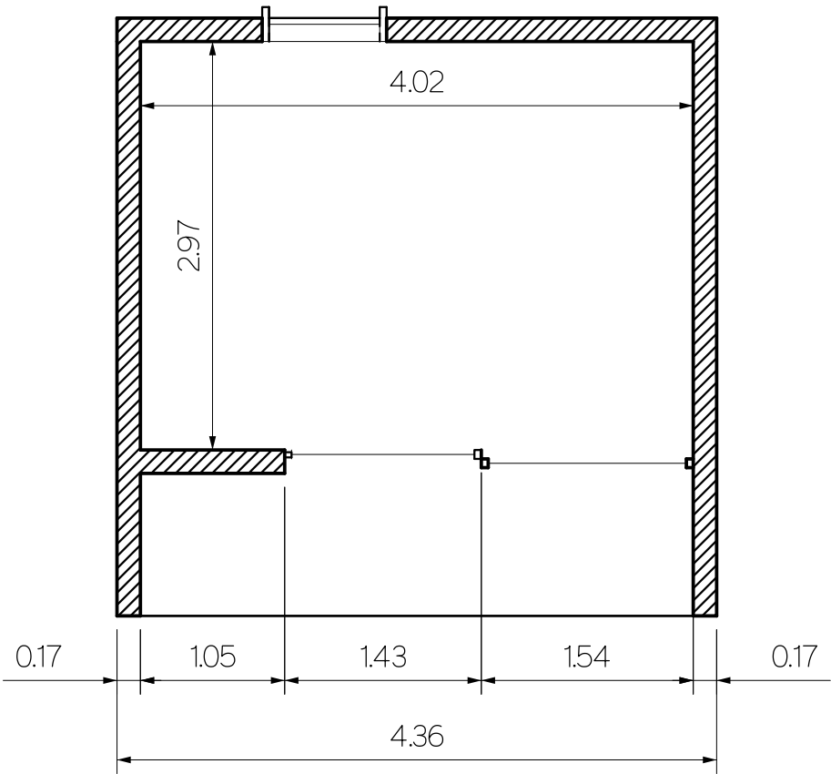
Planta Térrea
