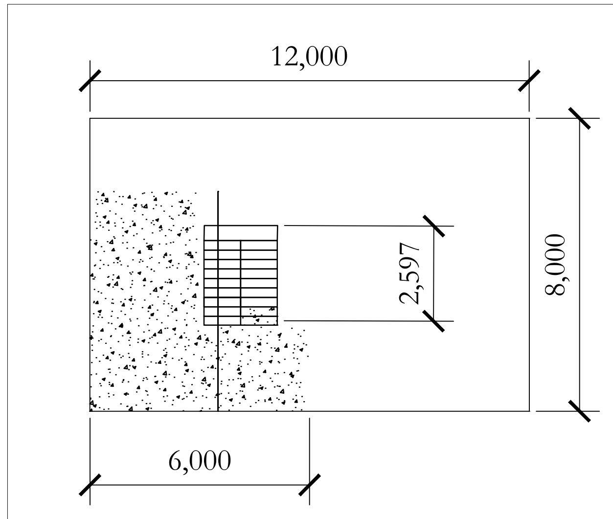
Corte Horizontal 1:100
