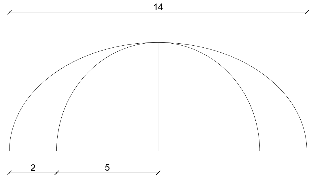
Alçado Lateral 1:100
