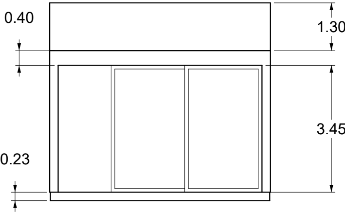
Alçado Sul
