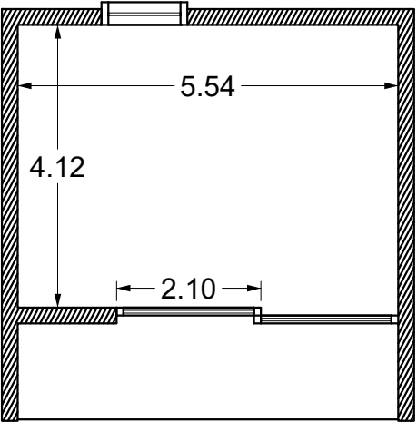
Planta Térrea
