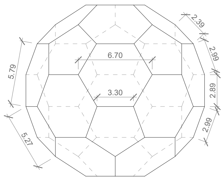
ALÇADO FRONTAL
