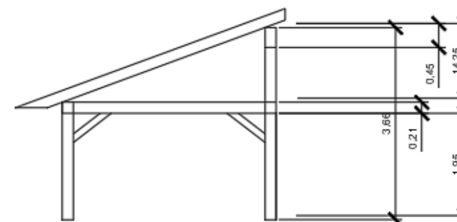
ALÇADO LATERAL COTADO, ESCALA 1:100
