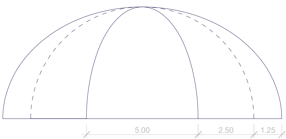
ALÇADO FRONTAL
