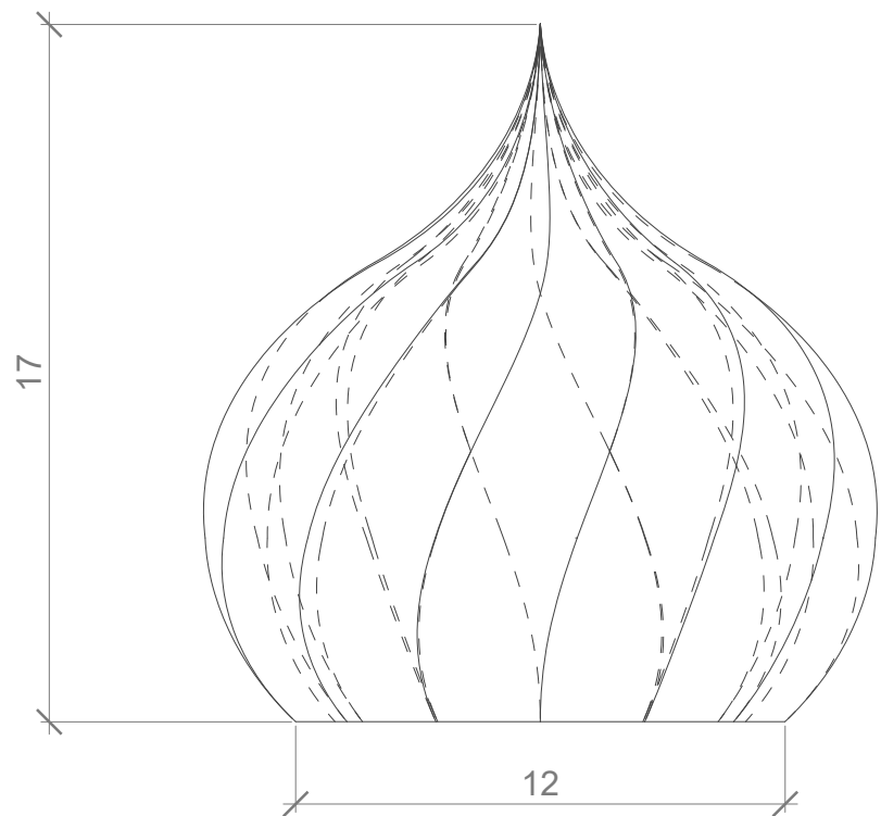
ALÇADO FRONTAL
