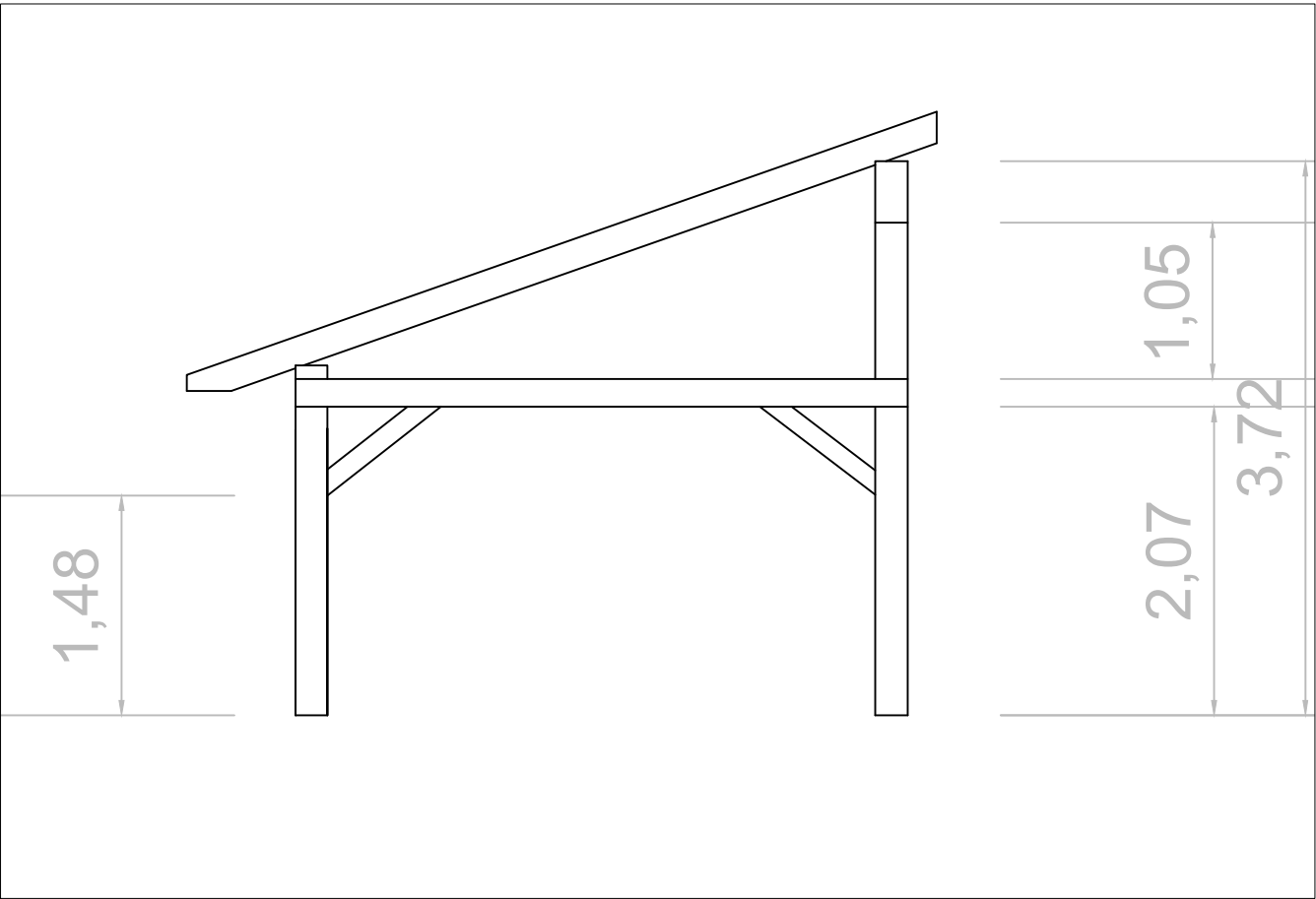
Alçado 1:50
