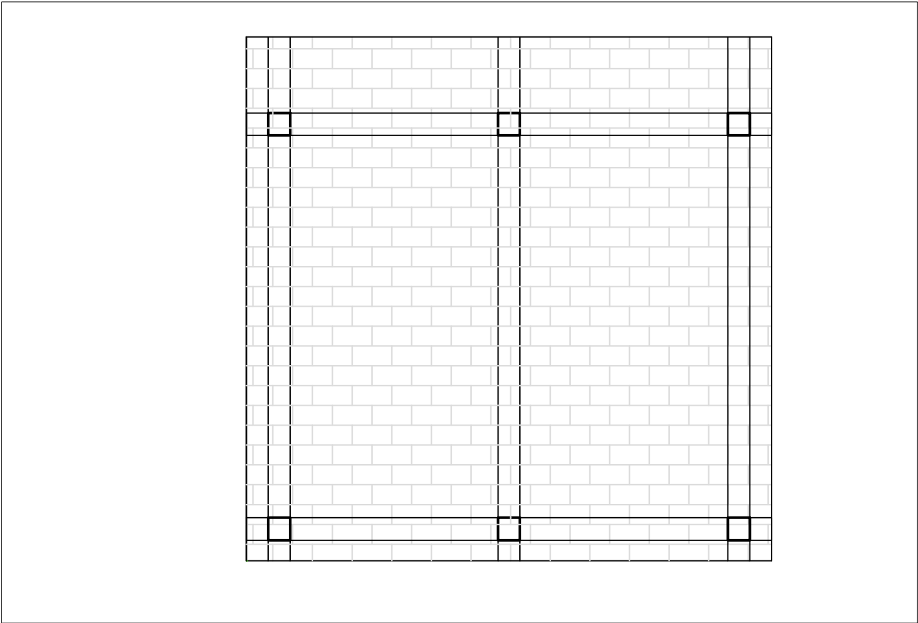
Planta 1:50
