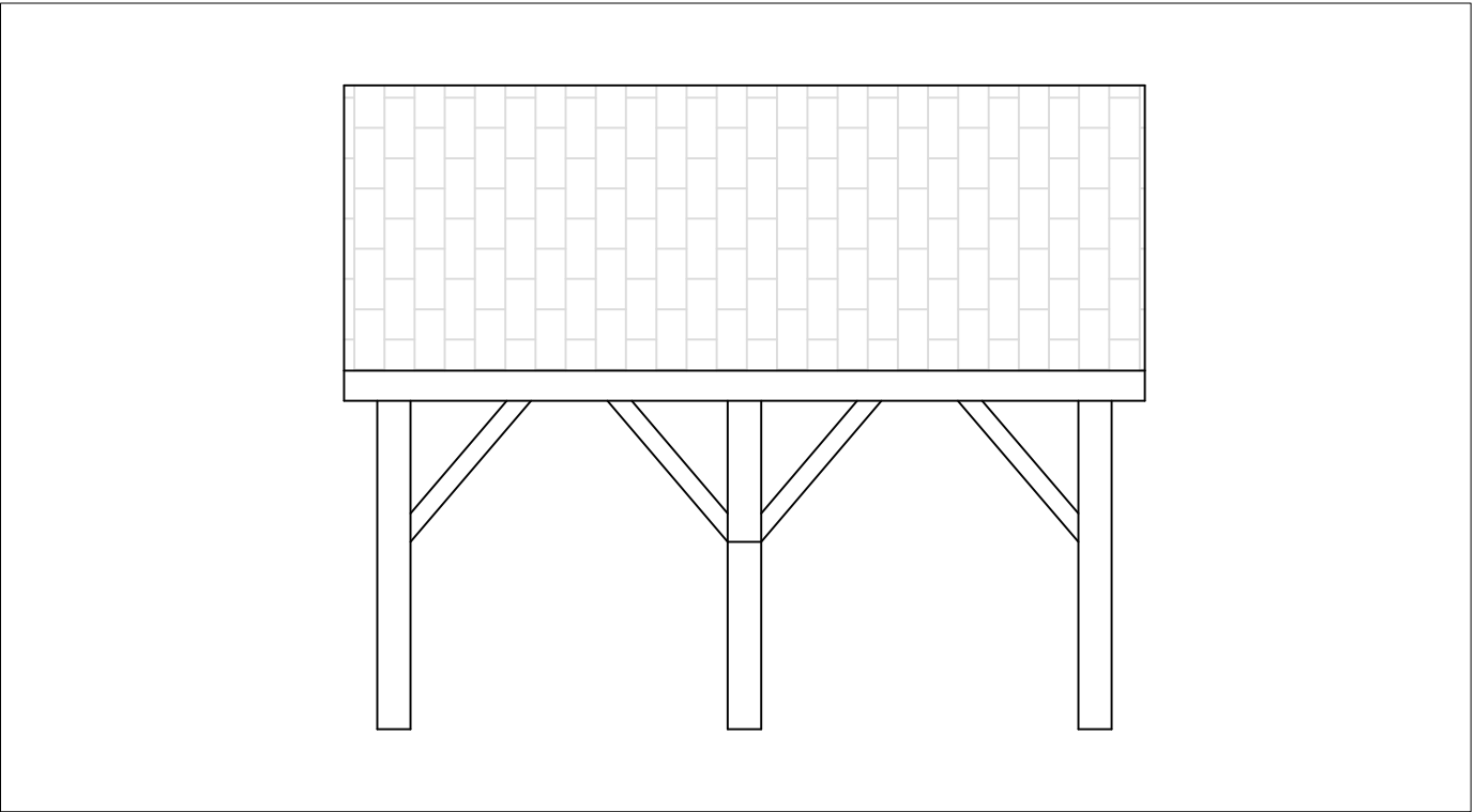
Alçado 1:50
