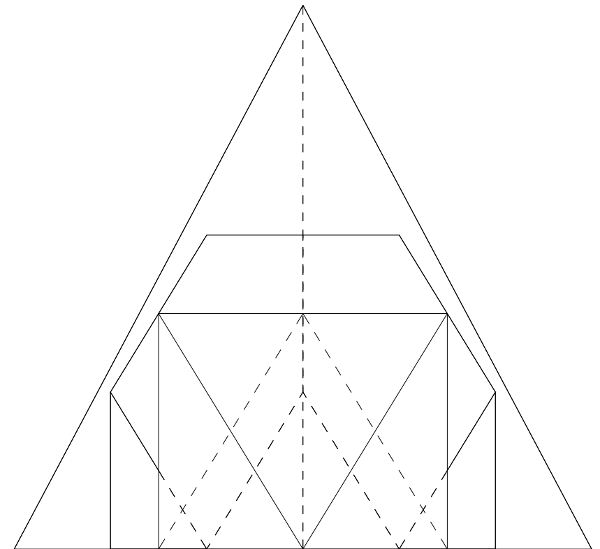
Alçado Lateral Esc 1:6
