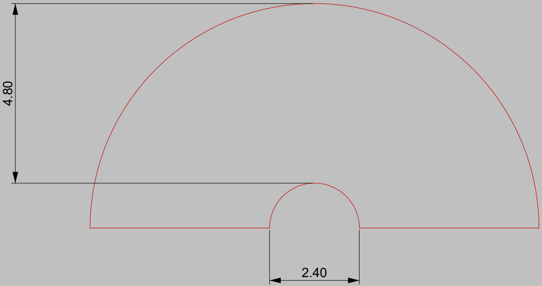
Planta esc. 1:1
