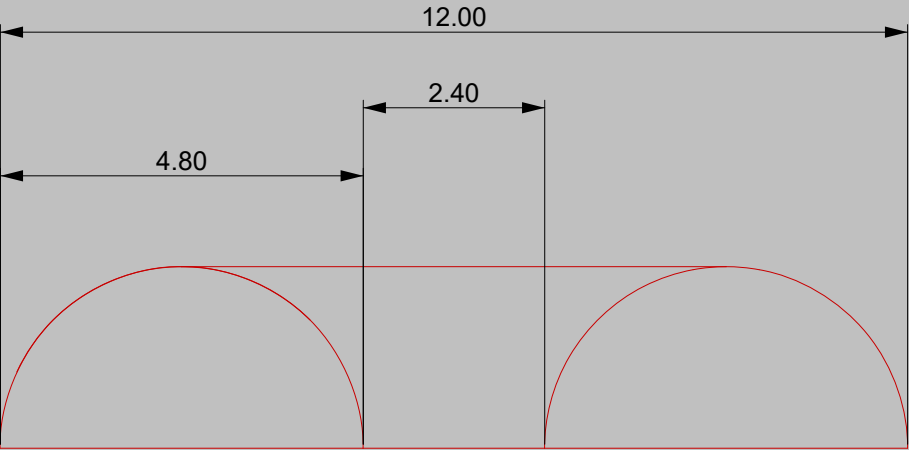
Alçado Frontal esc. 1:1
