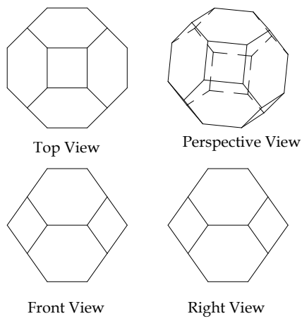
OCTAEDRO TRUNCADO
