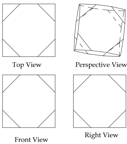
CUBO TRUNCADO
