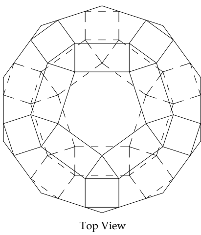
ROMBICOSIDODECAEDRO
