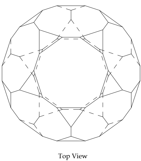
DODECAEDRO TRUNCADO
