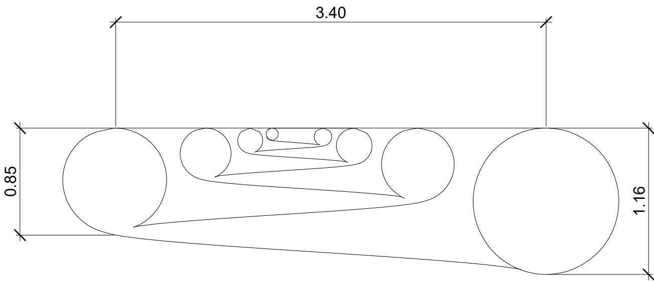
Alçado Frontal
