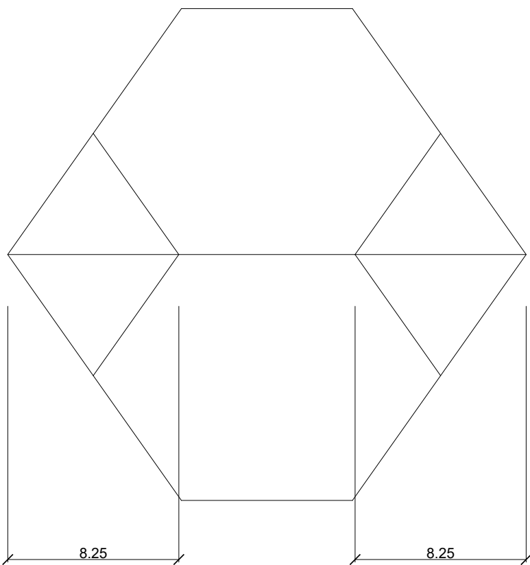
Alçado Lateral Dtº Esc. 1/1
