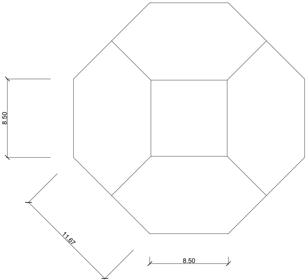
Planta Esc. 1/1
